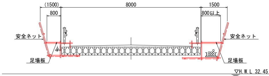
側部吊足場
