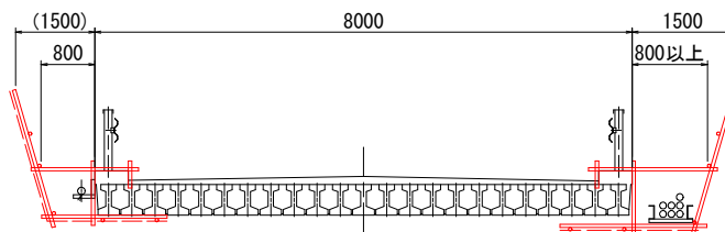
側部吊足場
