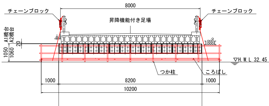
側部吊足場
