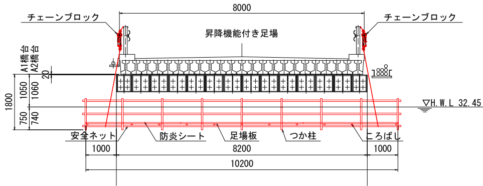
側部吊足場
