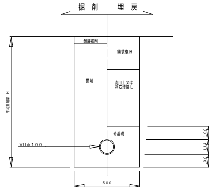
土工断面図 S = 1 : 10
