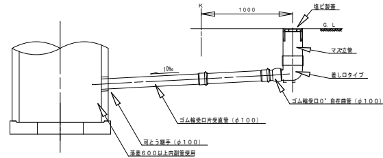
土工断面図 S = 1 : 10
